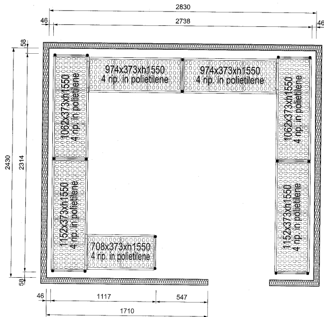
Boven aanzicht
